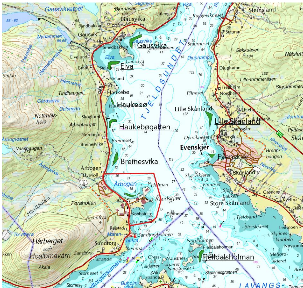
Figur 1. De potensielle ålegraslokalitetene som ble undersøkt er vist med grønne polygon. Understrekte navn viser lokalitetsnavn brukt i denne rapporten. Lokaliteten som ble registret i 2016 er innenfor planområdet (rød heltrukken linje). Lille Skånland utgikk i rekartleggingen 2019.
