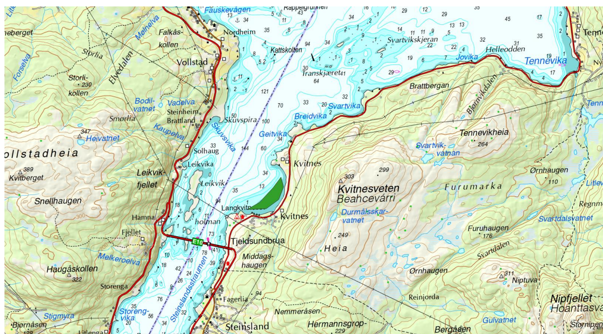
Figur 2. Grønt polygon markerer undersøkelsesområdet som ble lagt til som følge av lokalkunnskap. Området er Kvitnesbukta nord for Tjeldsundbrua.
