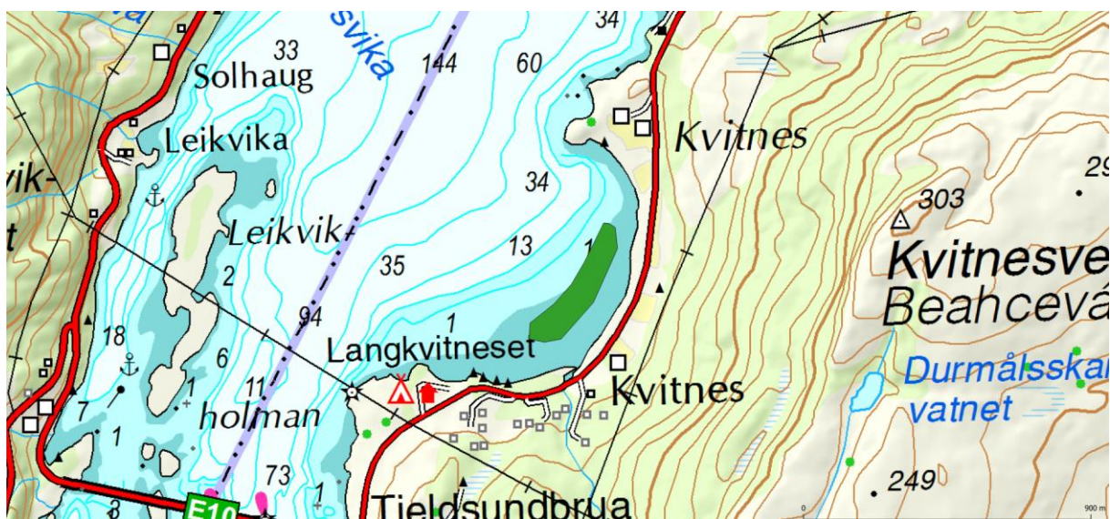
Figur 3. Grønt polygon viser avgrensning av registrert ålegraseng ved Kvitnes.
